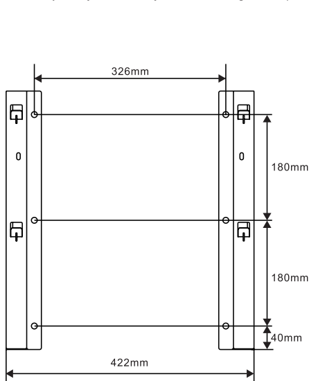
Rysunek wymiarowy uniwersalnego uchwytu dla innych modeli
