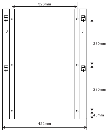
Rysunek wymiarowy dedykowanego uchwytu dla KS LB 48-100
